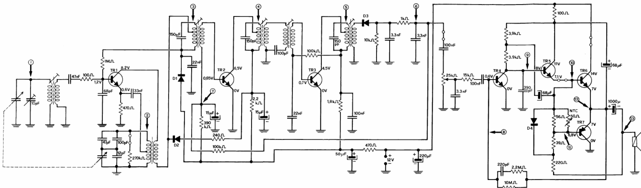
Tavola III - Schema elettrico di ricevitore per onde medie (Philips, mod. 22AN181). I numeri inseriti in cerchietti indicano i punti del circuito da cui sono prelevati i segnali riprodotti negli oscillogrammi.
